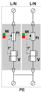
V: 高压敏电阻 Ft: 热熔断 t: 热脱扣机构 MI: 失效指示
