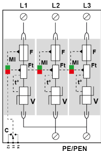
V: 高能压敏电阻 Ft: 热熔断 t: 热脱扣机构 MI: 失效指示
